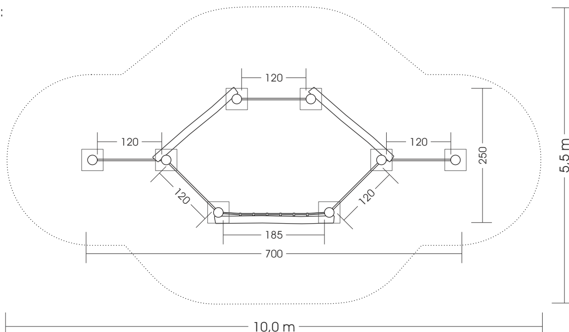
Draufsicht:
